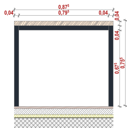
NO_MI-08 prerez b 1:20
