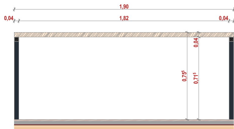
NO_MI-07 prerez a 1:20
