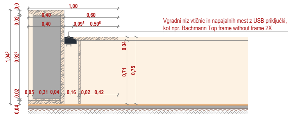
NO_MI-04 prerez C 1:25
