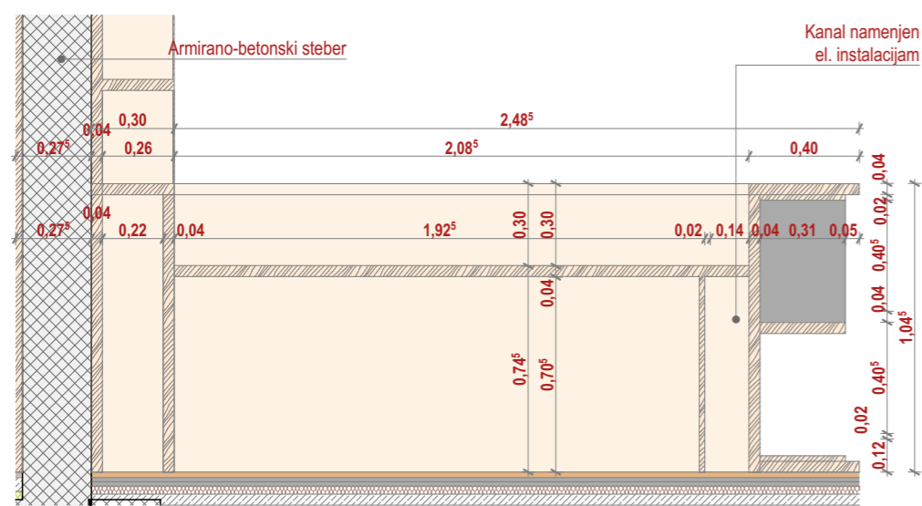
NO_MI-04 prerez b 1:25
