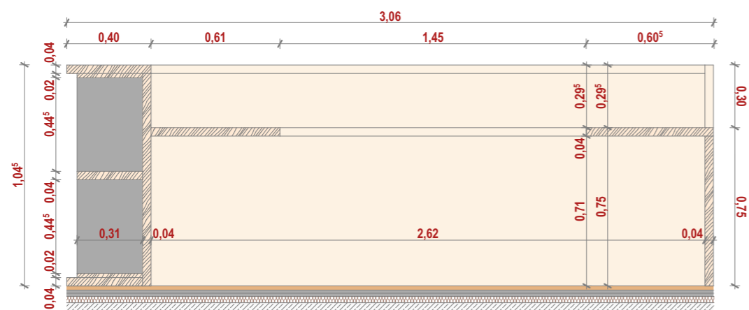
NO_MI-04 prerez a 1:25
