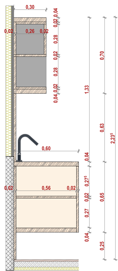
NO_PT-01 Prerez a 1:20
