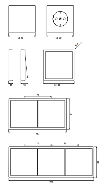
Primer vtičnice kot npr. jung LS 990 in Metal, v Antracitni barvi
