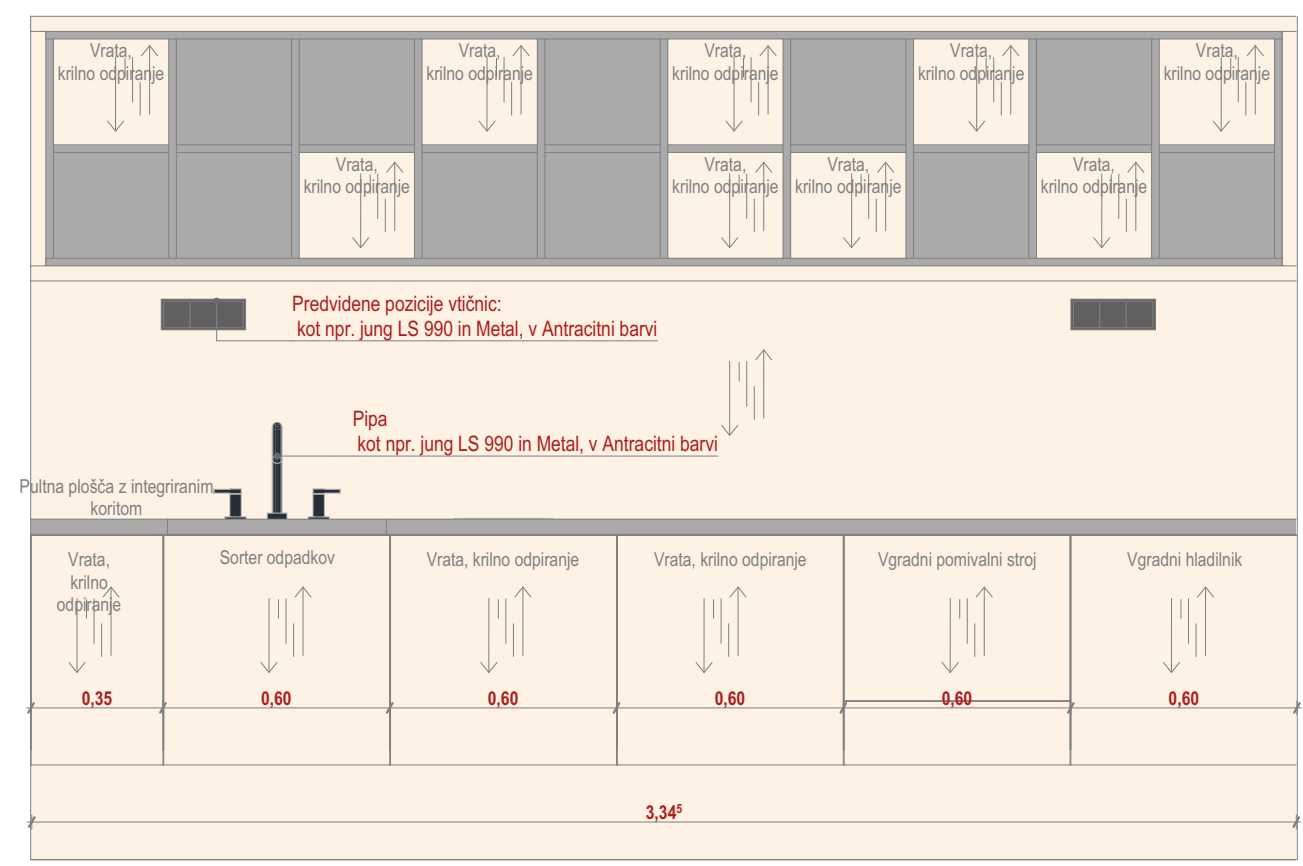
NO_PT-01 pogled 1:20
