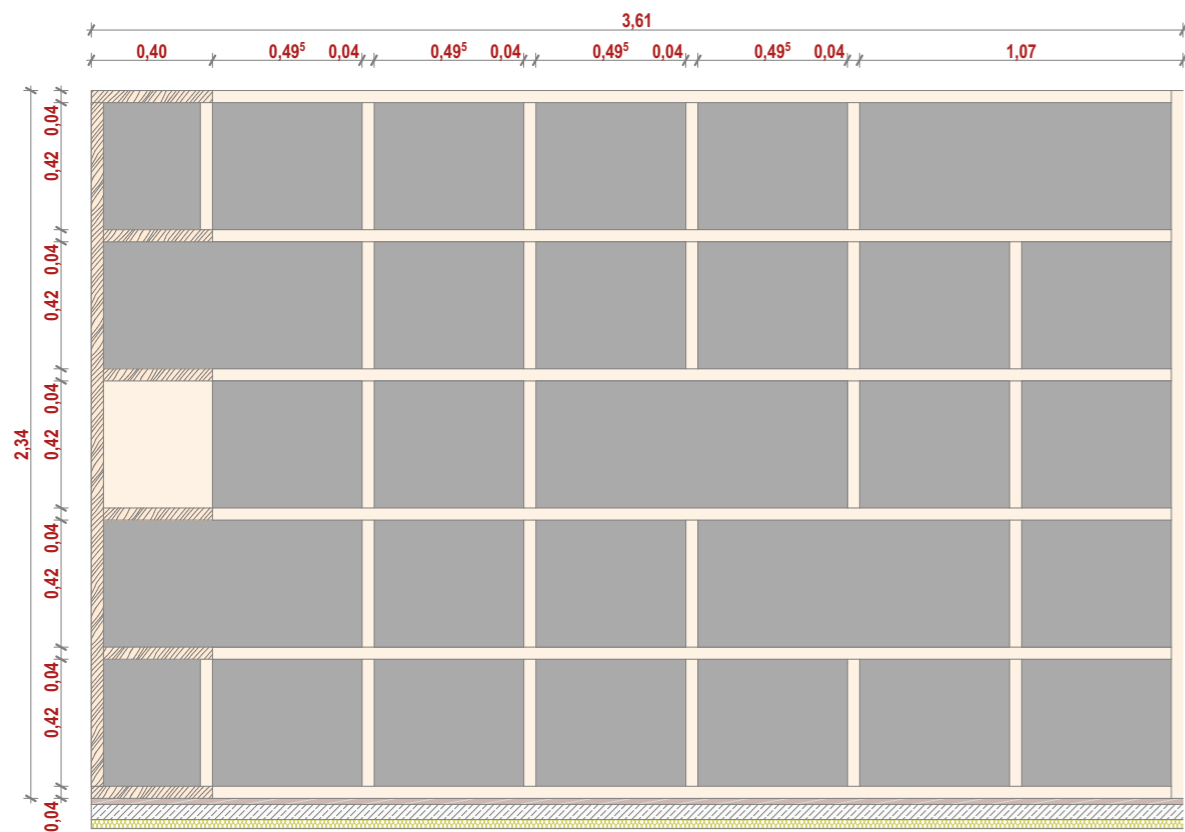
NO_OM-02 pogled 2 1:25
