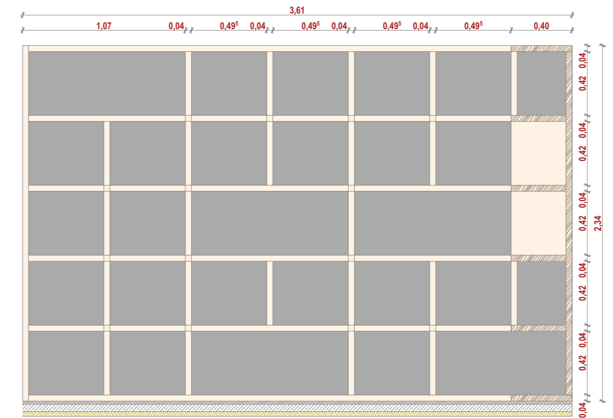
NO_OM-02 pogled 3 1:25
