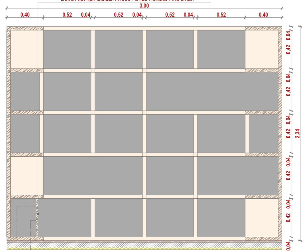
NO_OM-02 pogled 1 1:25
