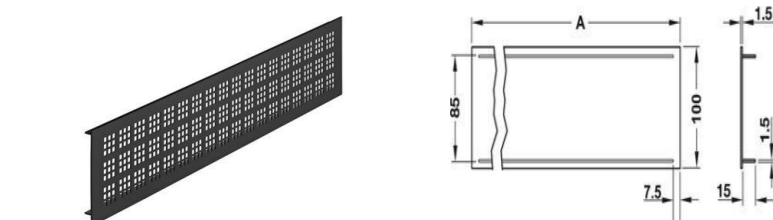
Primer prezračevalne rešetke
