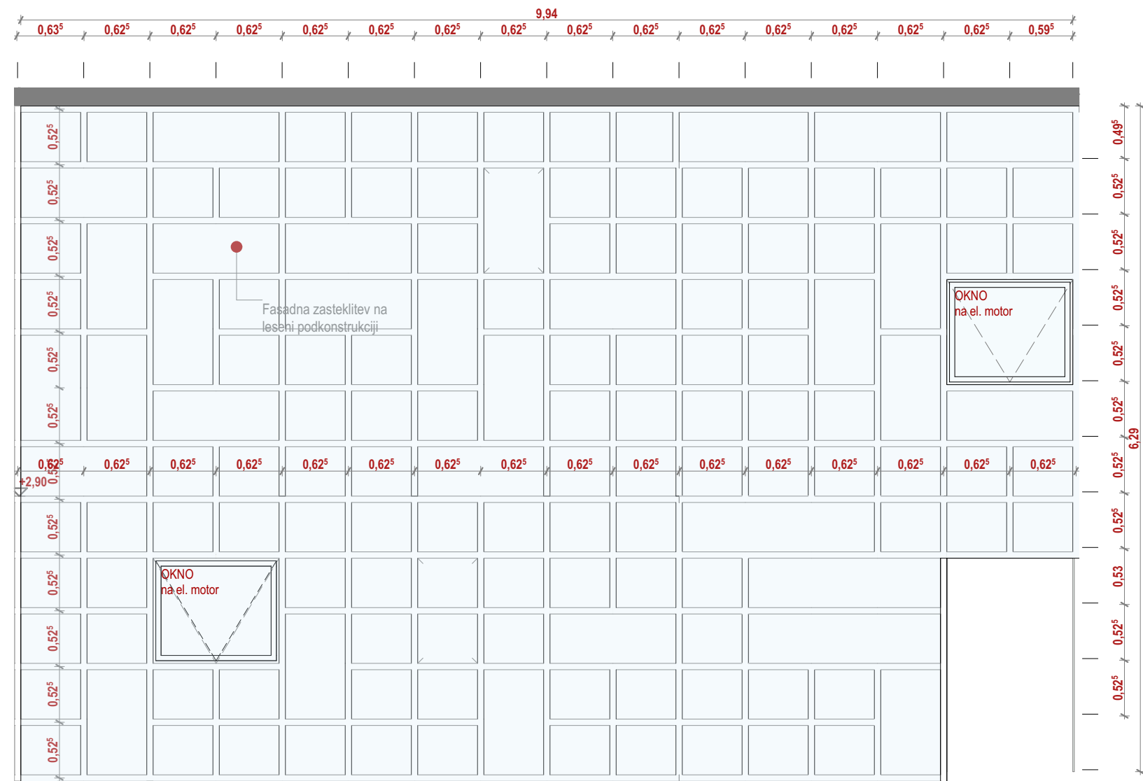
Steklarski detajli SD-01 1:50
