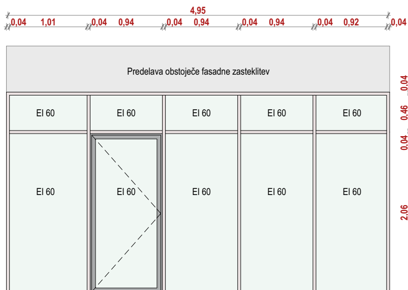
Steklarski detajli SDI-01/EI60 1:50
