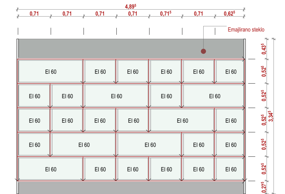
Steklarski detajli SD-03 1:50
