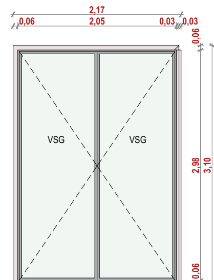
Steklarski detajli SDI-03 1:50
