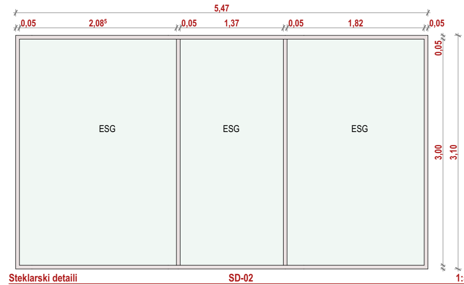
Steklarski detajli SD-02 1:50
