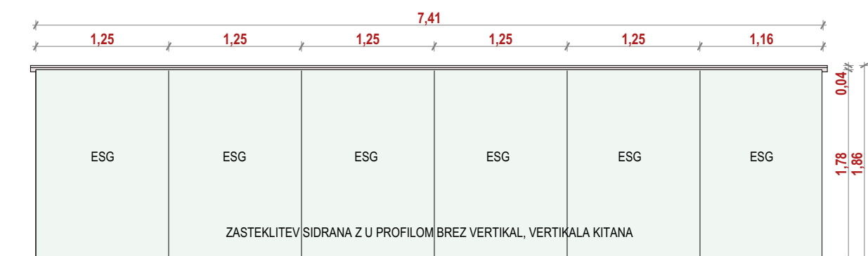
Steklarski detajli SDI-04 1:50
